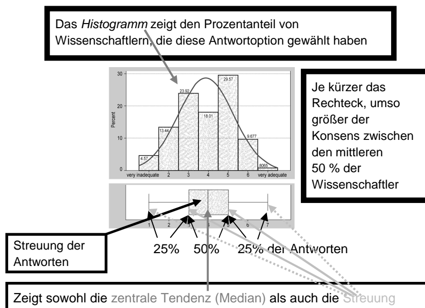
Abbildung 1. Boxplots
